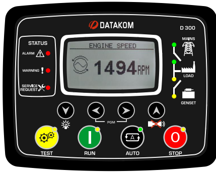
KONTROL CİHAZI
