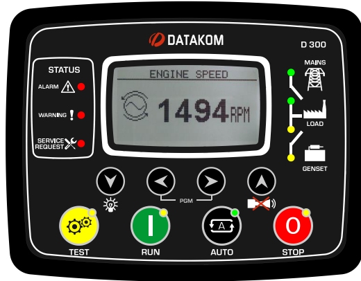
KONTROL CİHAZI
