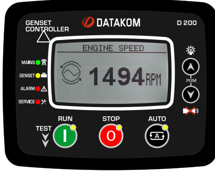
KONTROL CİHAZI
