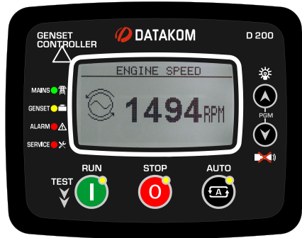
KONTROL CİHAZI
