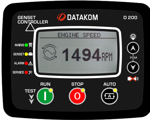
KONTROL CİHAZI
